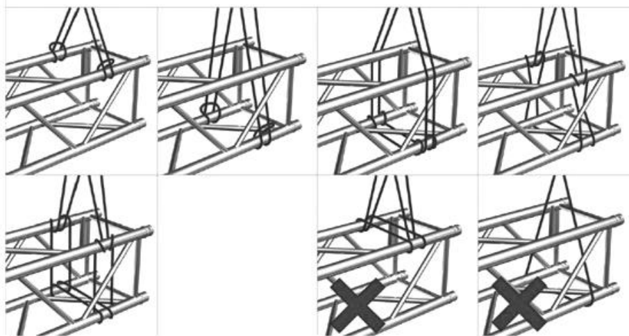
图1 编织吊索吊挂桁架方式
